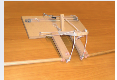
| Kelluvien johtojen mekaanisen liittimen malli
